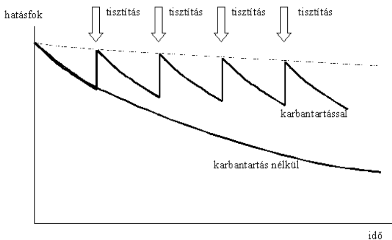
4.6. ábra. A lámpatestek avulása
