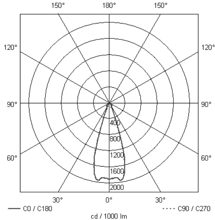
4.5/c. ábra. Forgásszimmetrikus fényvető fényeloszlása. Az ilyen lámpatest valamennyi C síkban felvett fényeloszlása azonos. A fény irányításának mértéke a fél- vagy tizedértékszöggel fejezhető ki. Erősen irányított fényvetők görbéjét polárkoordináták helyett derékszögű (Descartes) koordinátákban szokás megadni.
